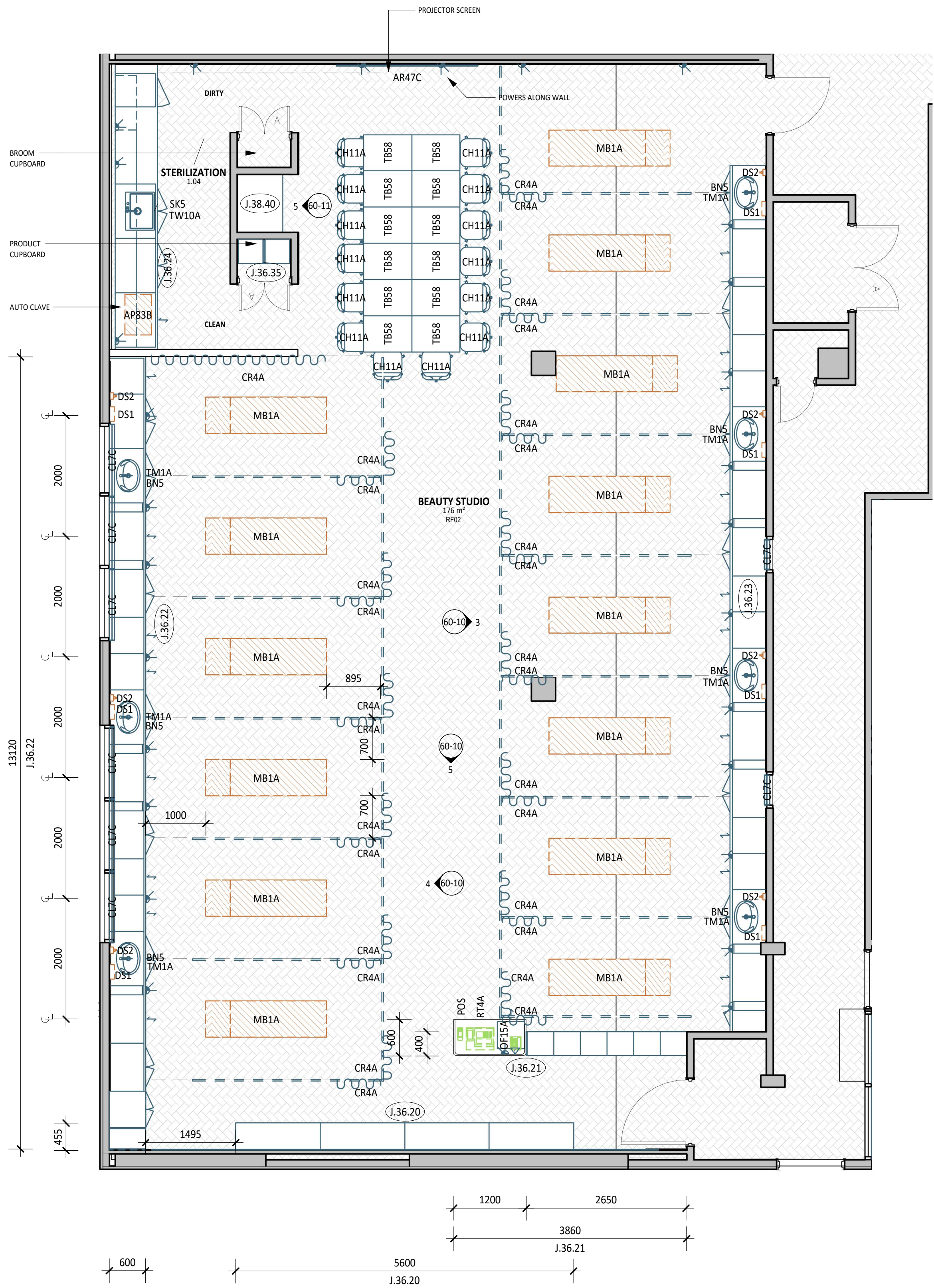
1 PLAN DETAIL 1 : 50
